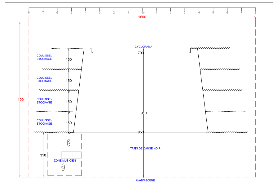
Plan d'implantation type à l'italienne
